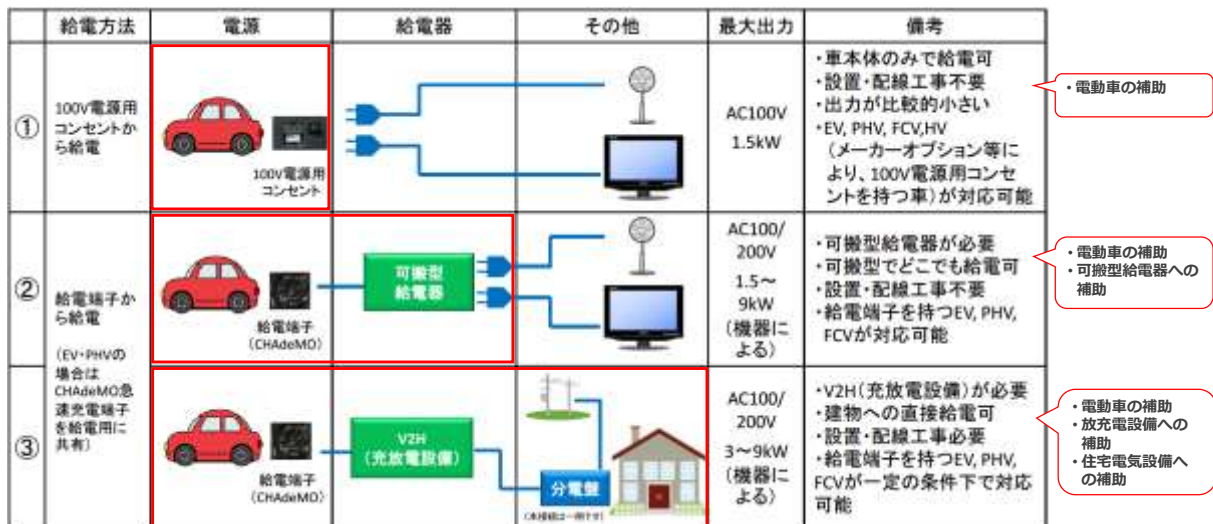
図 4-30 EV の電源活用に関するタイプ分け
