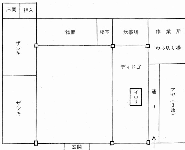
図6 事例6，天間館字柳平野田頭福之進氏宅
